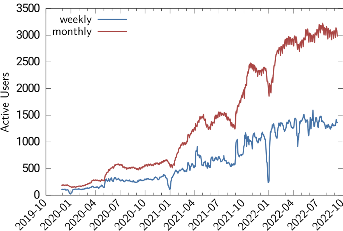
GitLab
