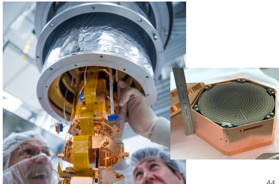
SuperCDMS detector
